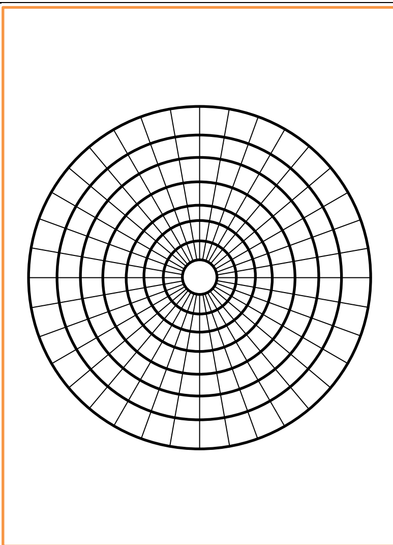
Рис. 2. Линии параллелей южного полушарий картографической сетки перспективной центральной полярной проекции
